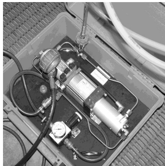
Bild: Gasbooster
